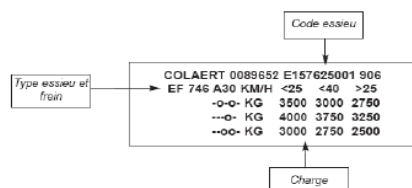
PLAQUETTE D'IDENTIFICATION ESSIEU (Soudée sur le carré d'essieu)
